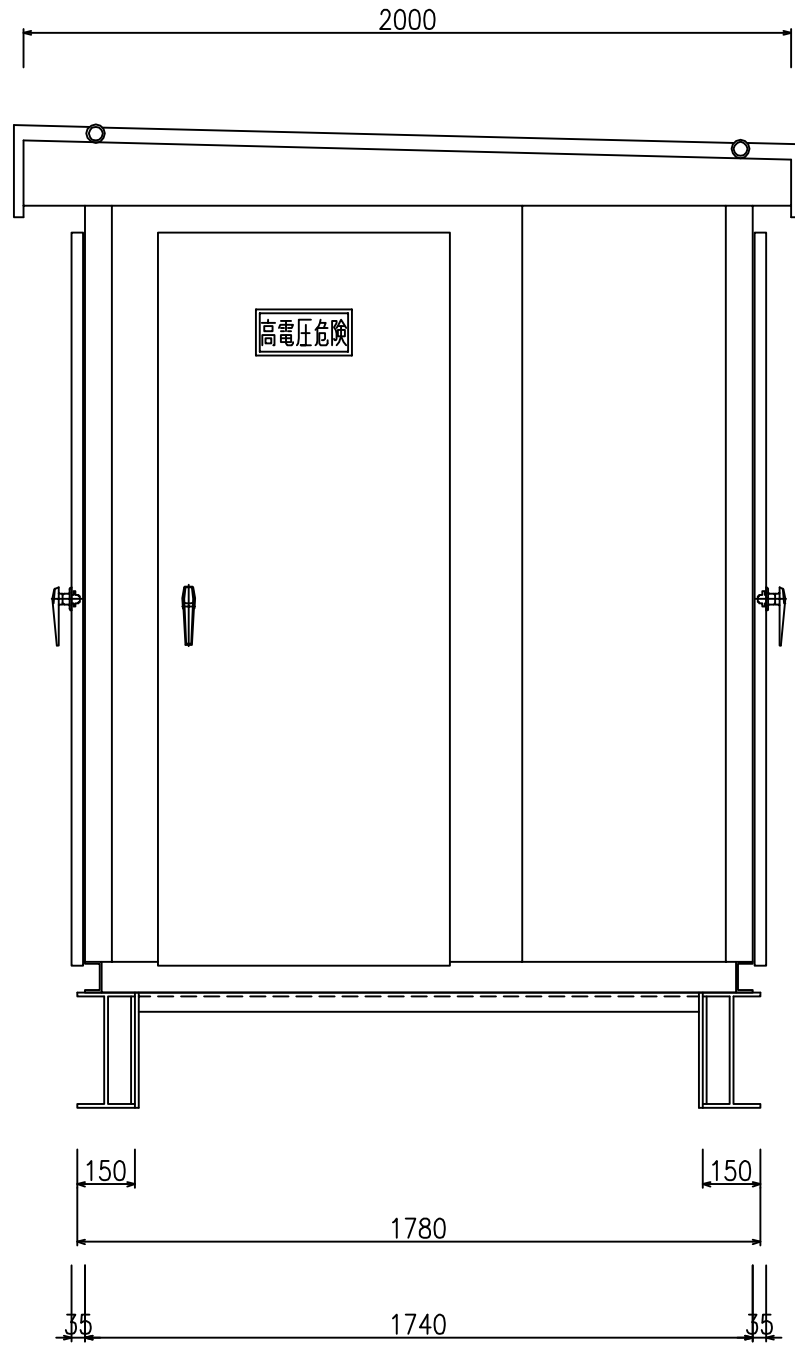
側面図
