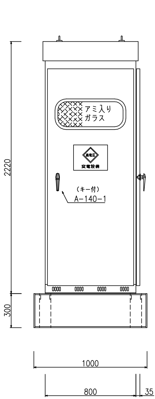
正面図
