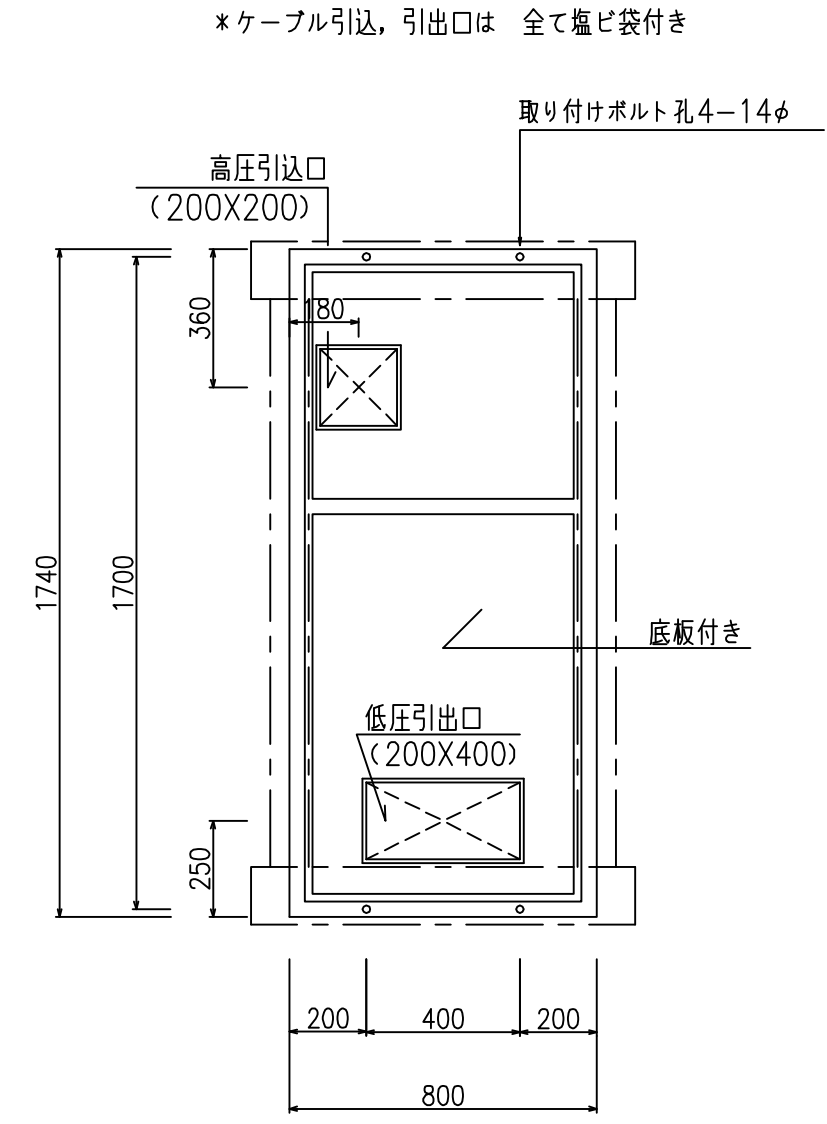
基礎図
